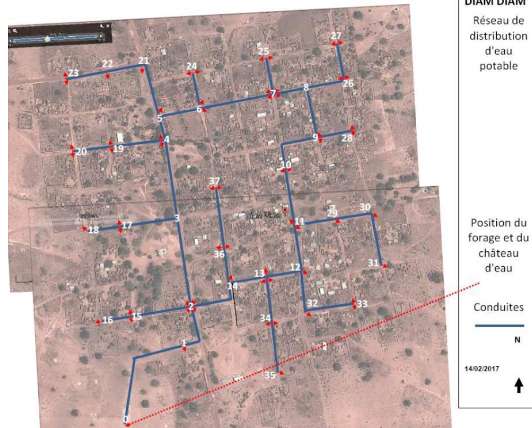
Schéma d'aménagement des branchements privés phase 2
