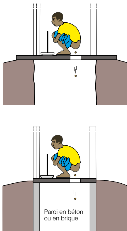
Figure 25. Les dalles bien soutenues peuvent être plus petites
