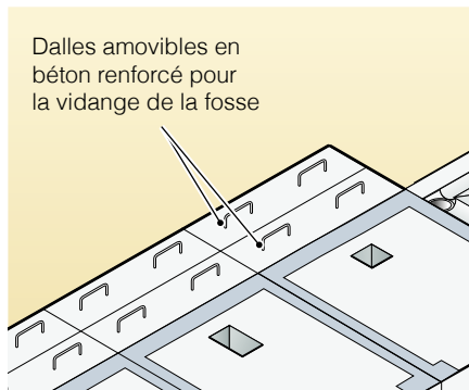
Figure 15. Les poignées facilitent le retrait de la dalle
