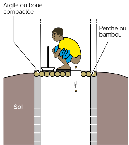
Figure 21. Une dalle est soutenue par des rondins, bâtons ou bambous avec de l'argile pour remplir les espaces
