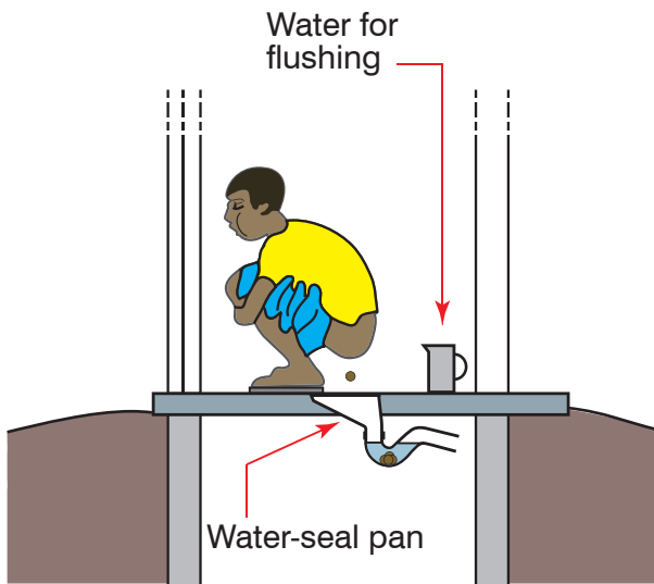
Figure 7. A pour-flush pan
