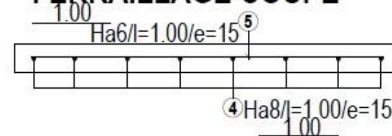
FERRAILLAGE COUPE
