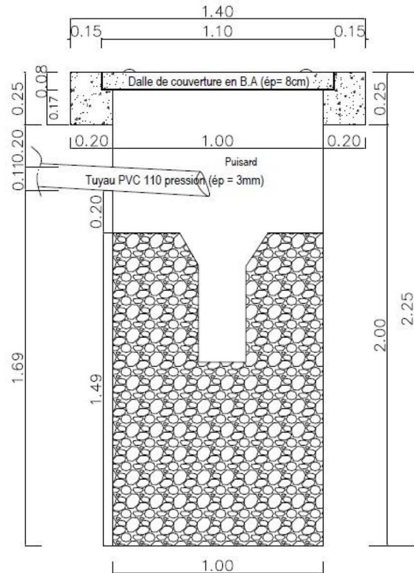
COUPE B-B
