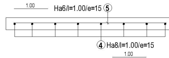
FERRAILLAGE COUPE
