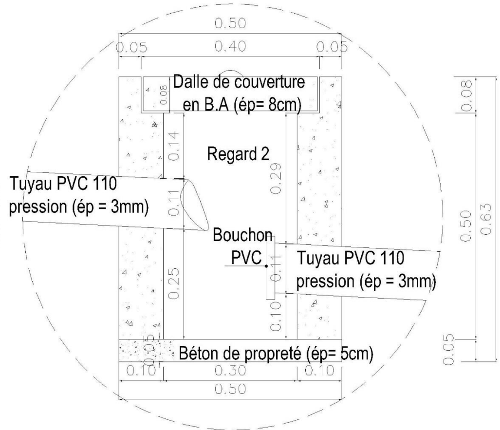
COUPE A-A
