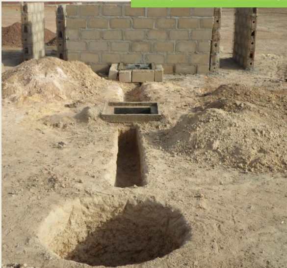
Chenal d'évacuation équipé de 2 regards et conduisant à un puisard de 2m de profondeur rempli de moellons
