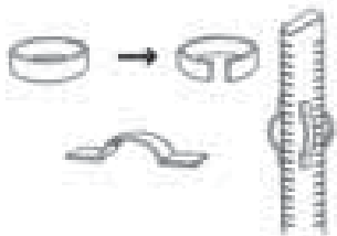
Centreurs artisanaux attachés à la crépine
