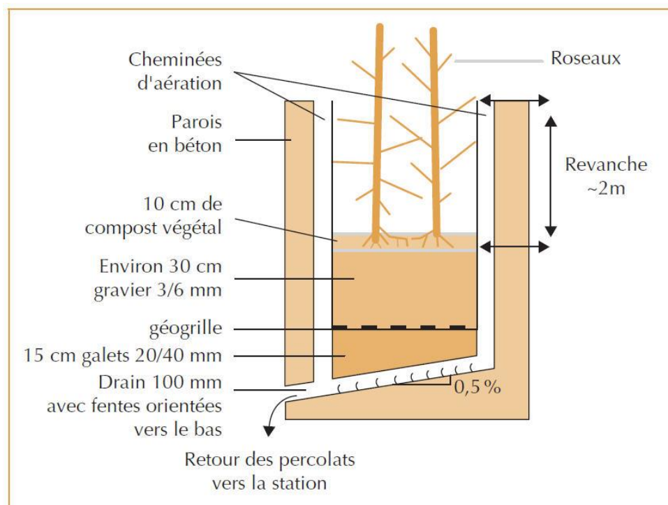
Figure 8 : Coupe schématique de lit de séchage planté de roseaux
