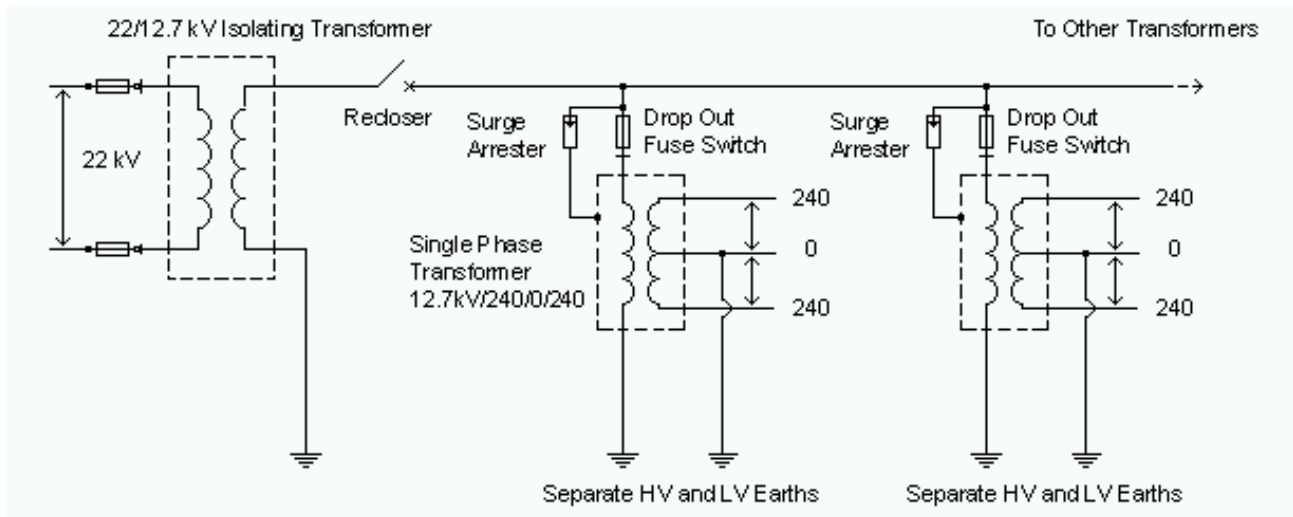
Fig. 8: Schéma électrique d'une ligne SWER
