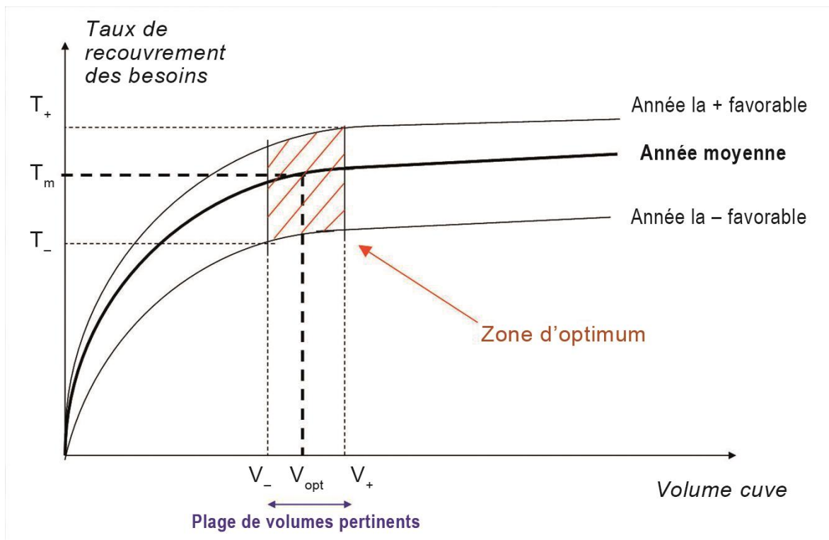
Figure 5 : Zone d'optimum de d finition du volume d'une cuve
