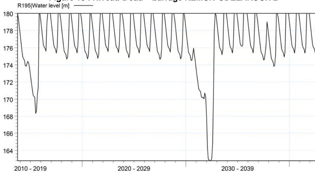
Figure 20 : Niveau d'eau – barrage N'GBEHOUEDO 2
