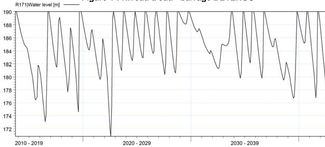
Figure 2 : Niveau d'eau - barrage VOSSA
