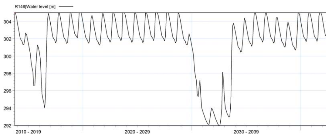
Figure 4 : Niveau d'eau - barrage DONGA
