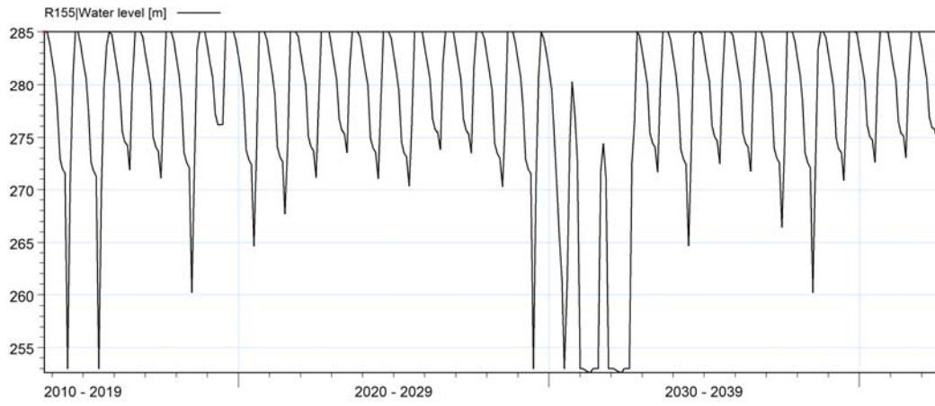
Figure 10 : Niveau d'eau - barrage IGBO-MACRO
