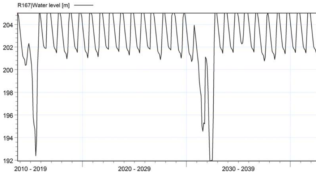
Figure 19 : Niveau d'eau – barrage KEMON-ODELAKOUN 2
