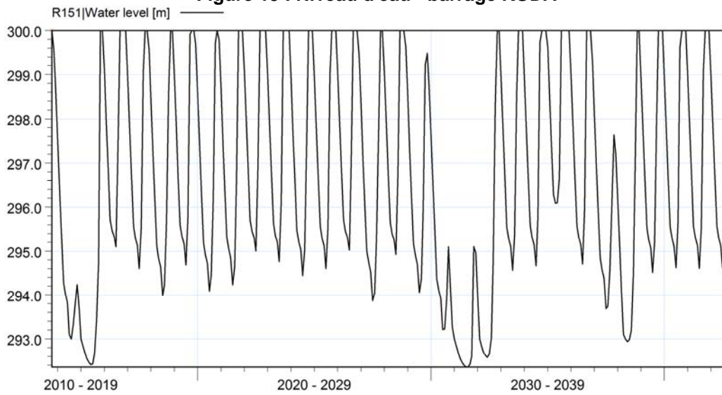
Figure 14 : Niveau d'eau - barrage TANDOU
