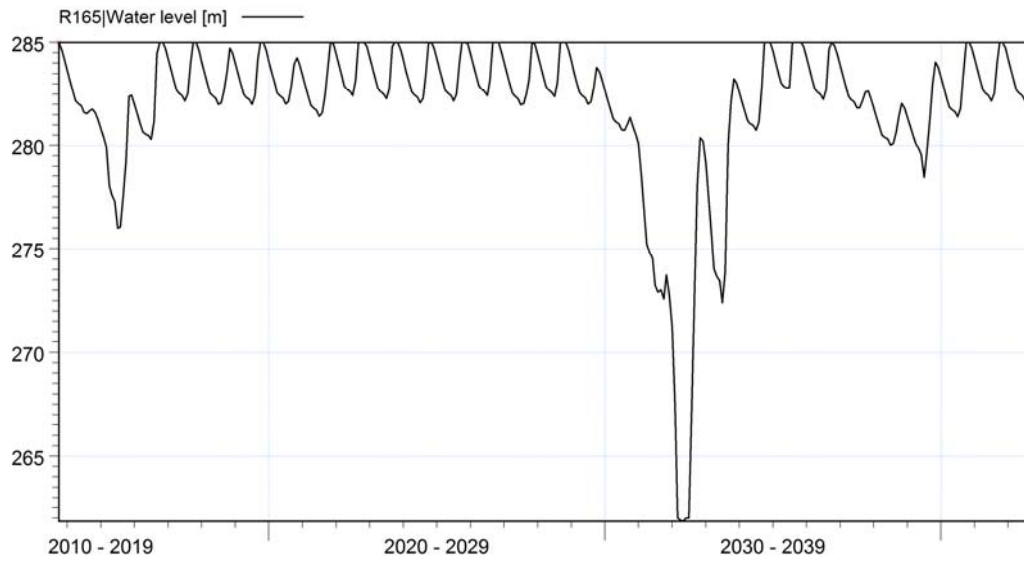
Figure 16 : Niveau d'eau – barrage BIGUINA 1
