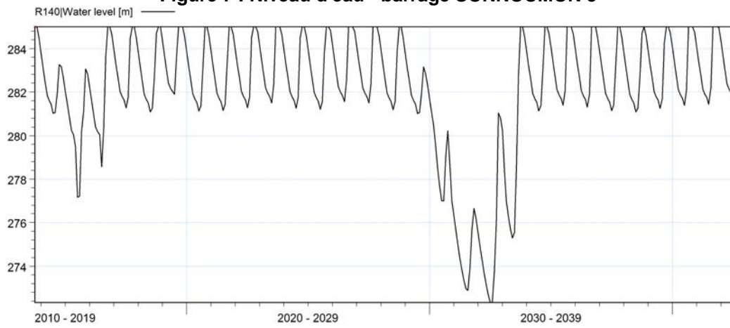
Figure 8 : Niveau d'eau - barrage TOUROU VI
