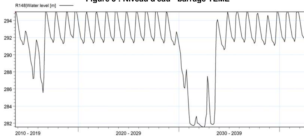
Figure 6 : Niveau d'eau - barrage SONNOUMON 2
