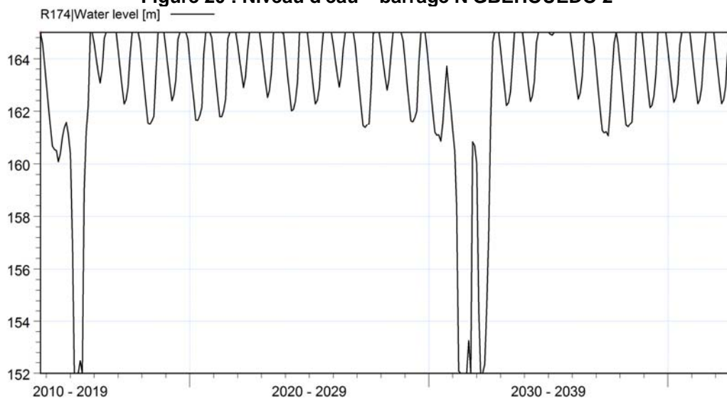
Figure 21 : Niveau d'eau – barrage AMOU
