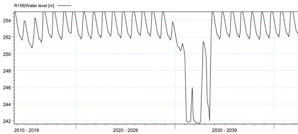
Figure 11 : Niveau d'eau - barrage DOGUE 1
