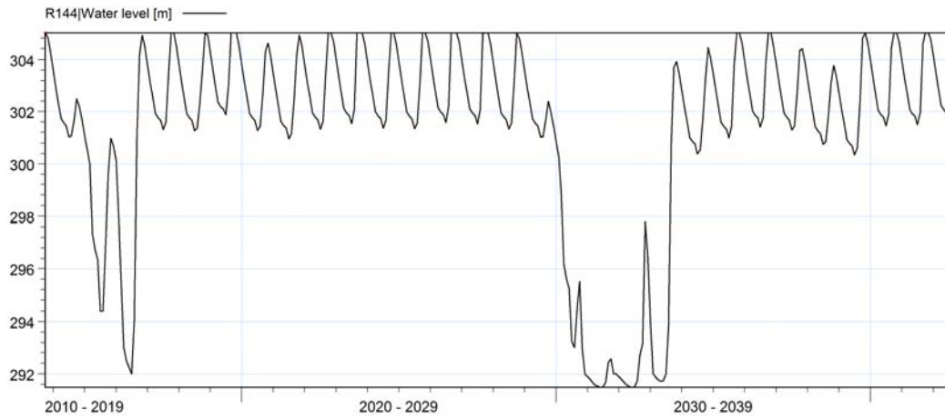
Figure 7 : Niveau d'eau - barrage SONNOUMON 3
