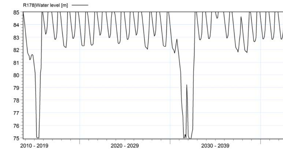
Figure 27 : Niveau d'eau – barrage KONKONDJI
