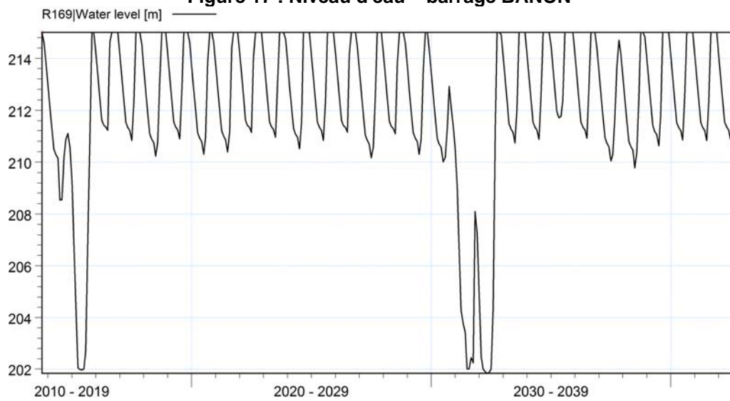
Figure 18 : Niveau d'eau – barrage KEMON-ODELAKOUN 1
