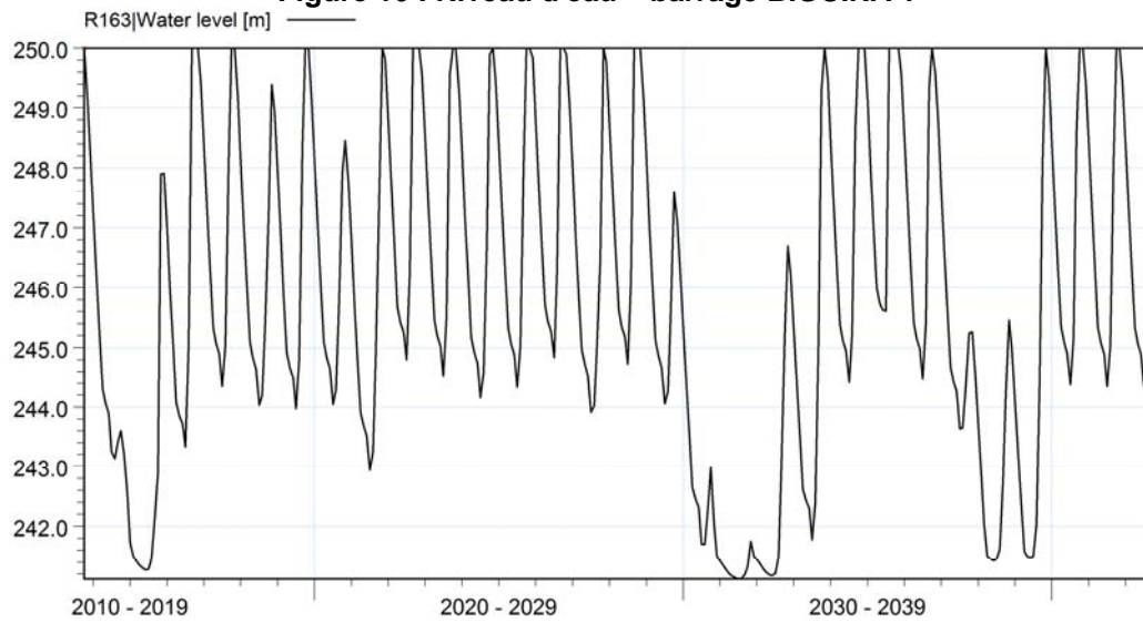
Figure 17 : Niveau d'eau – barrage BANON
