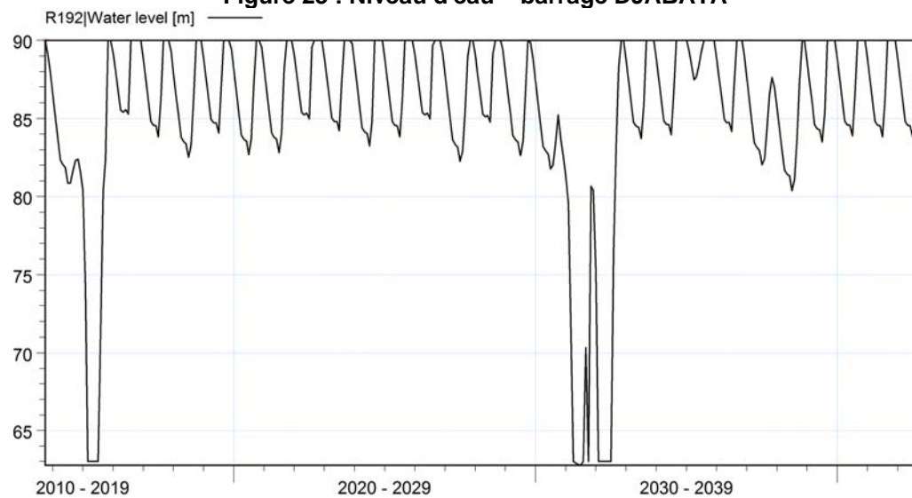
Figure 24 : Niveau d'eau – barrage IGBODJA
