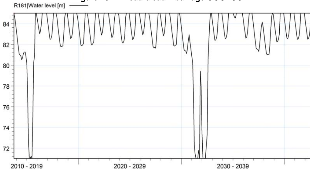
Figure 26 : Niveau d'eau – barrage GOBADA
