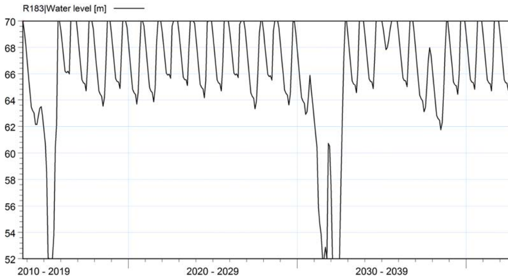
Figure 25 : Niveau d'eau – barrage GOUNSOE
