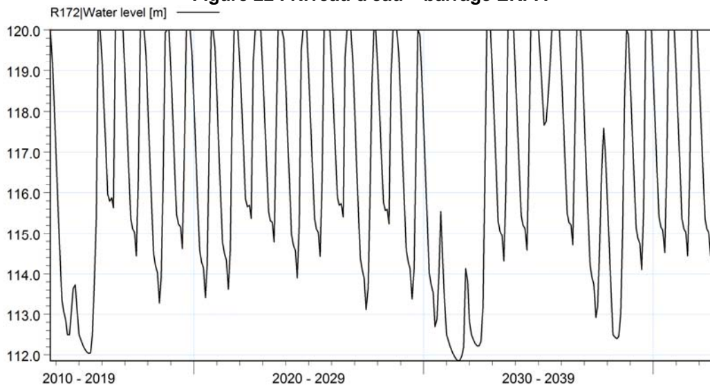
Figure 23 : Niveau d'eau – barrage DJABATA
