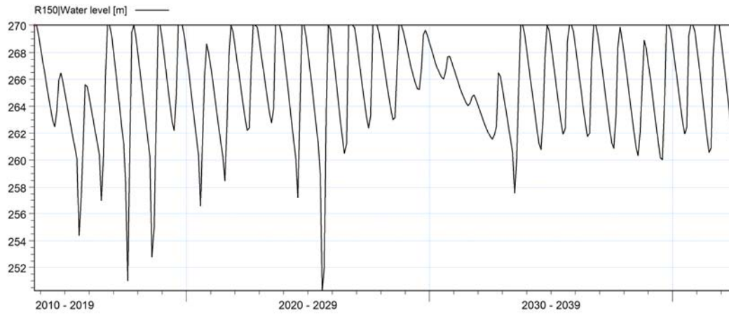
Figure 1 : Niveau d'eau - barrage BETEROU
