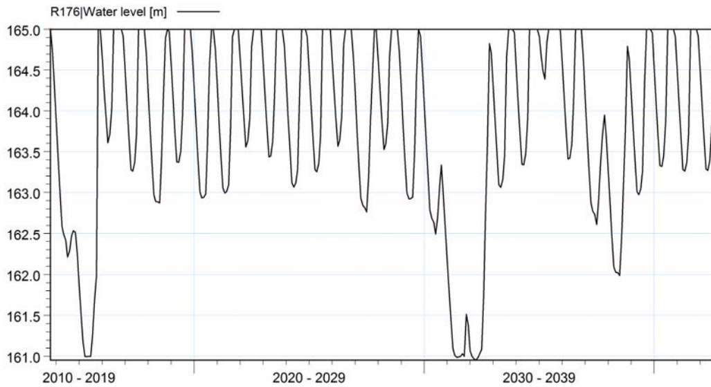
Figure 22 : Niveau d'eau – barrage EKPA
