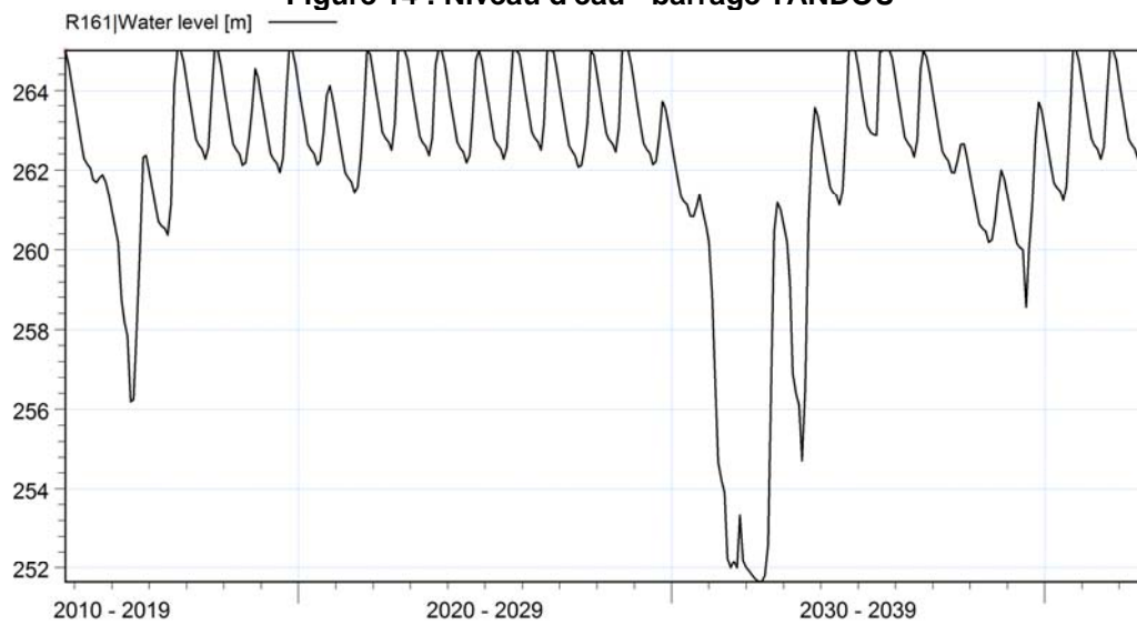
Figure 15 : Niveau d'eau – barrage IGBERE 2
