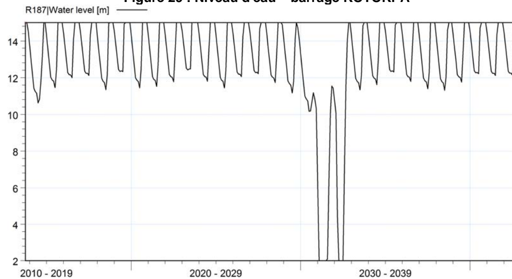
Figure 30 : Niveau d'eau – barrage GBOKOUTOU
