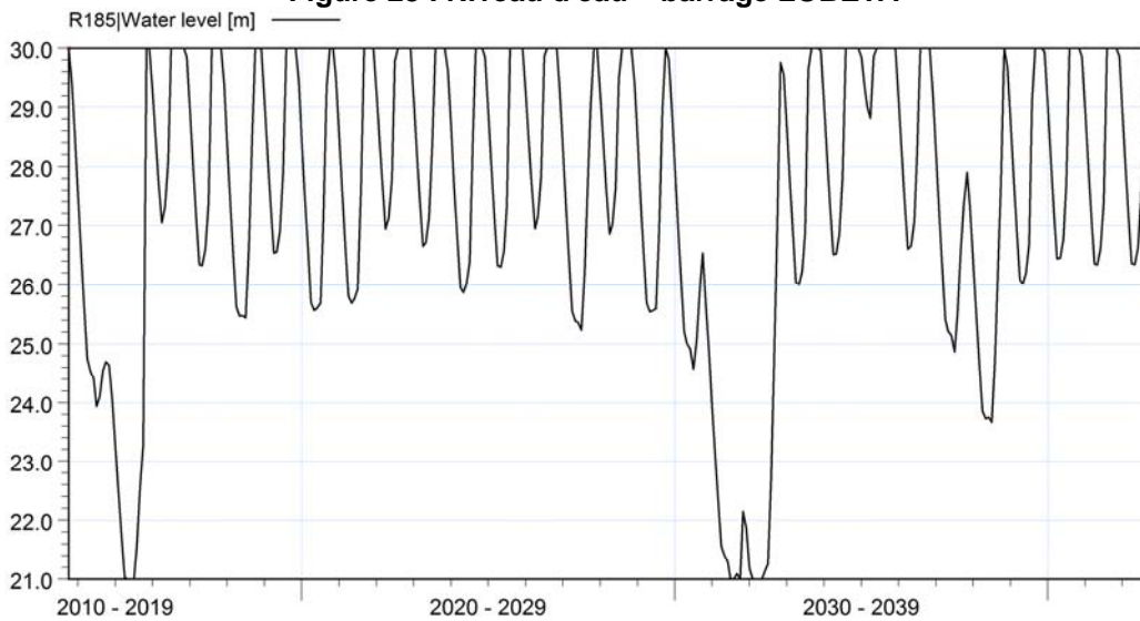
Figure 29 : Niveau d'eau – barrage KOTOKPA
