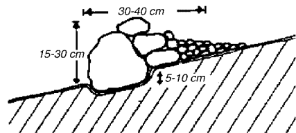
B: Coupe transversale
