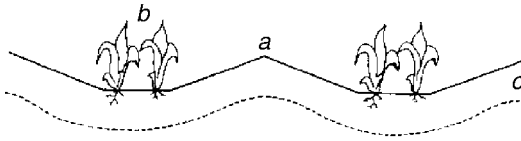
A: Microbassin sans mulching
