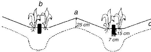
B: Microbassin avec mulching vertical
