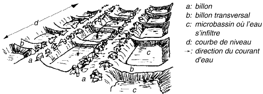
Figure 29 : Diguettes en damier légèrement inclinées par rapport à la courbe de niveau.
