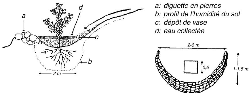
Figure 25 : Petite diguette semi-circulaire coupe transversale et vue aérienne.
