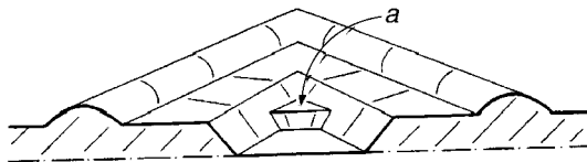
Figure 22 : Microbassins fermés (Critchley, 1991).
