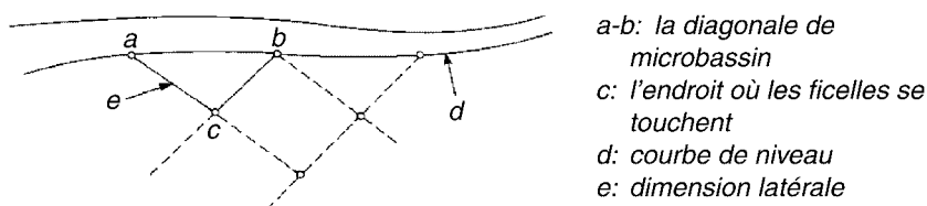
Figure 23 : Disposition des microbassins (Critchley, 1991).
