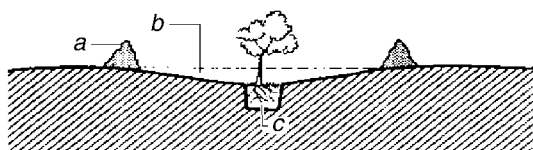
B: Coupe transversale
