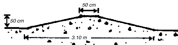
B: Coupe transversale d'une diguette plus grande (au 'fond' de la diguette)
