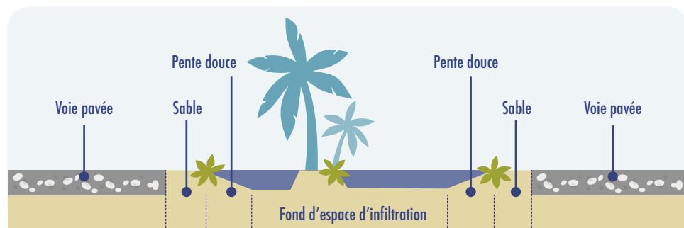
Figure 10. Projet de décaissement de la place et revêtement perméable périphérique
