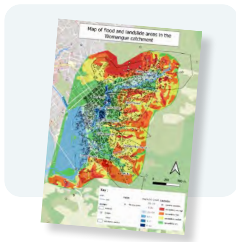
Figure 6. Cartes de zones inondables obtenues par modélisation hydraulique
