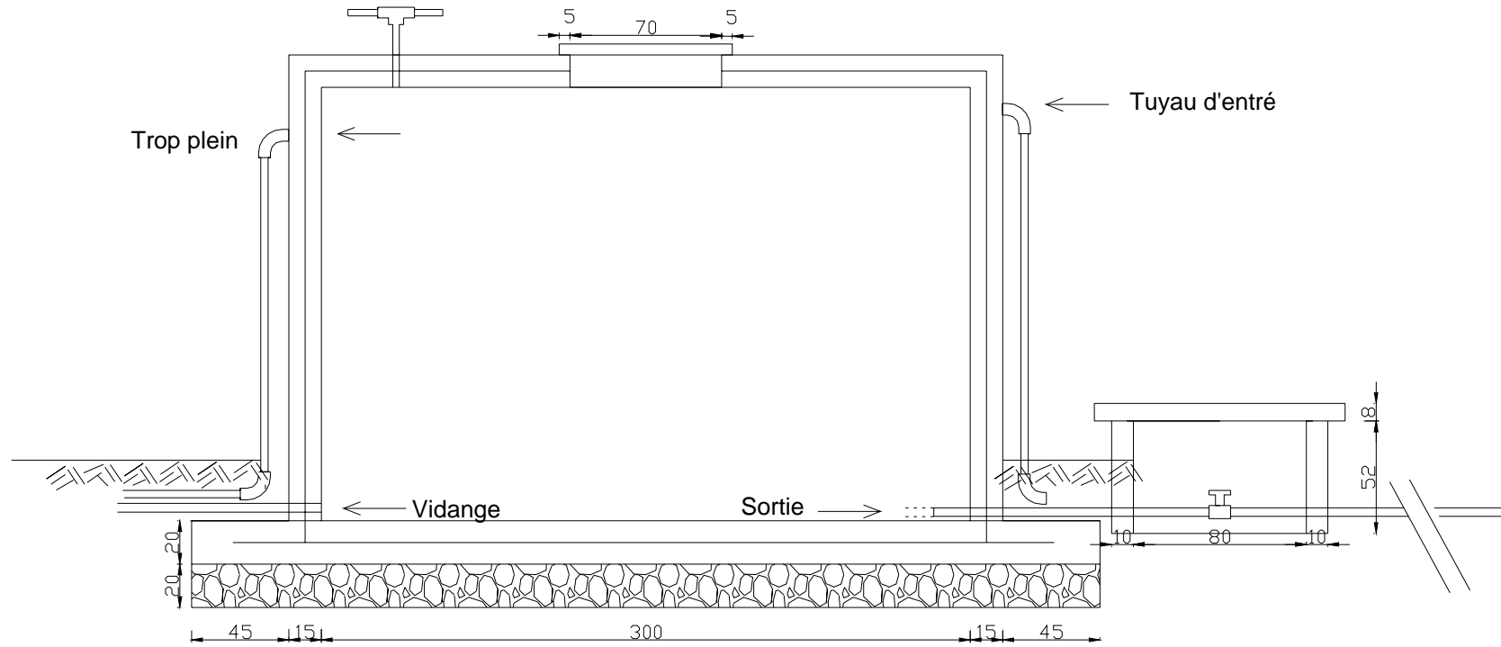
COUPE A-A
